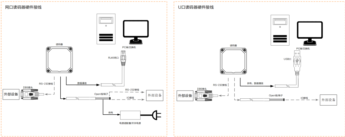
图 6-2 硬件接线
