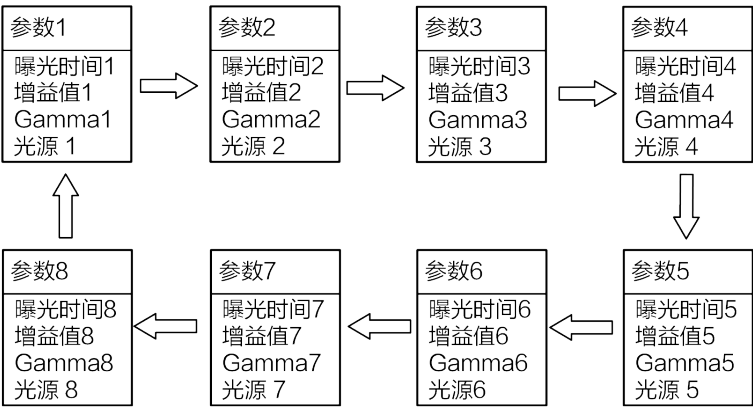
图 8-3 轮询示意图
