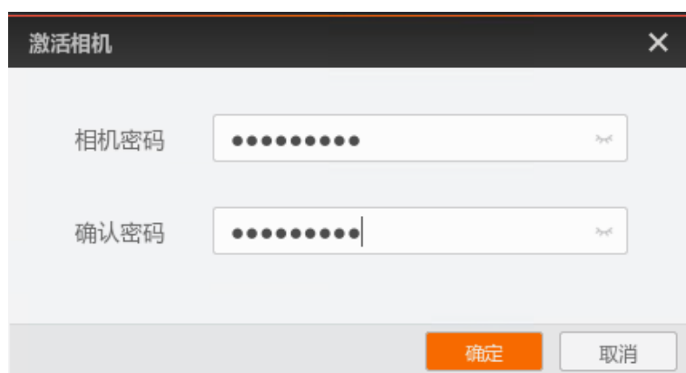
图 6-8 设置密码
