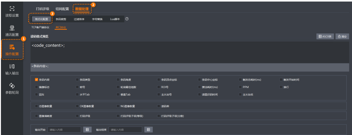
图 8-5 格式化配置
