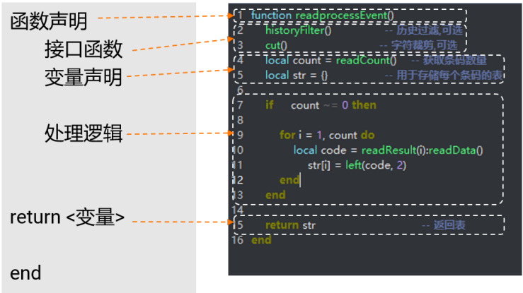
图 9-15 脚本结构
