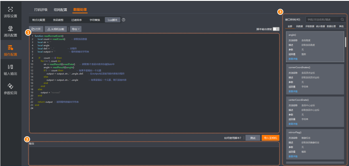
图 9-14 Lua 脚本
