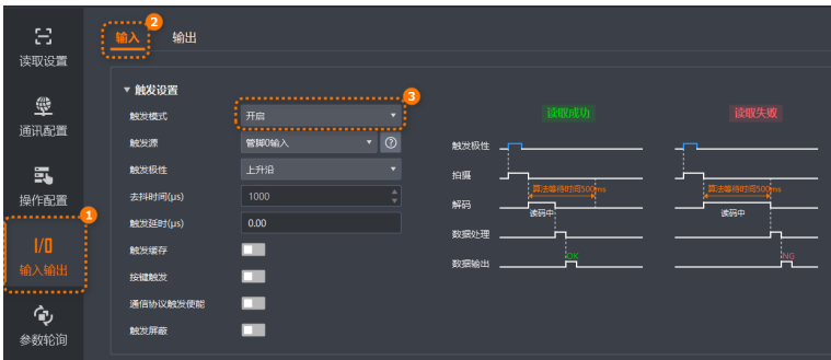
图 8-14 触发设置
