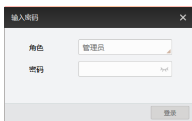
图 11-5 输入密码
