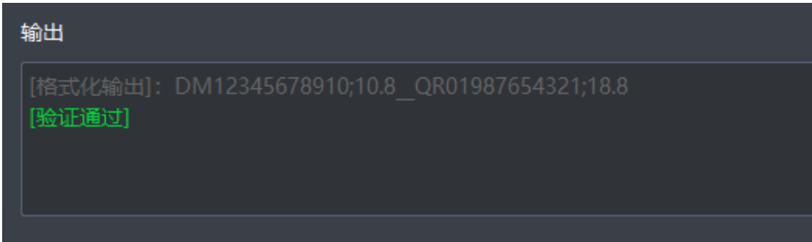
图 9-17 验证脚本
