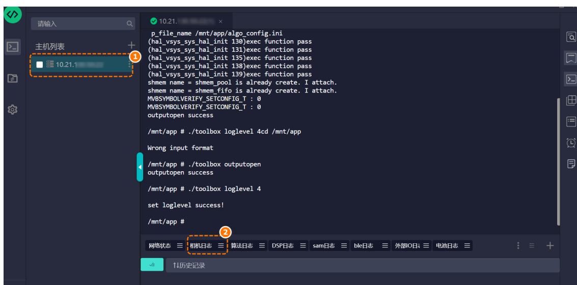
图 11-15 相机日志
