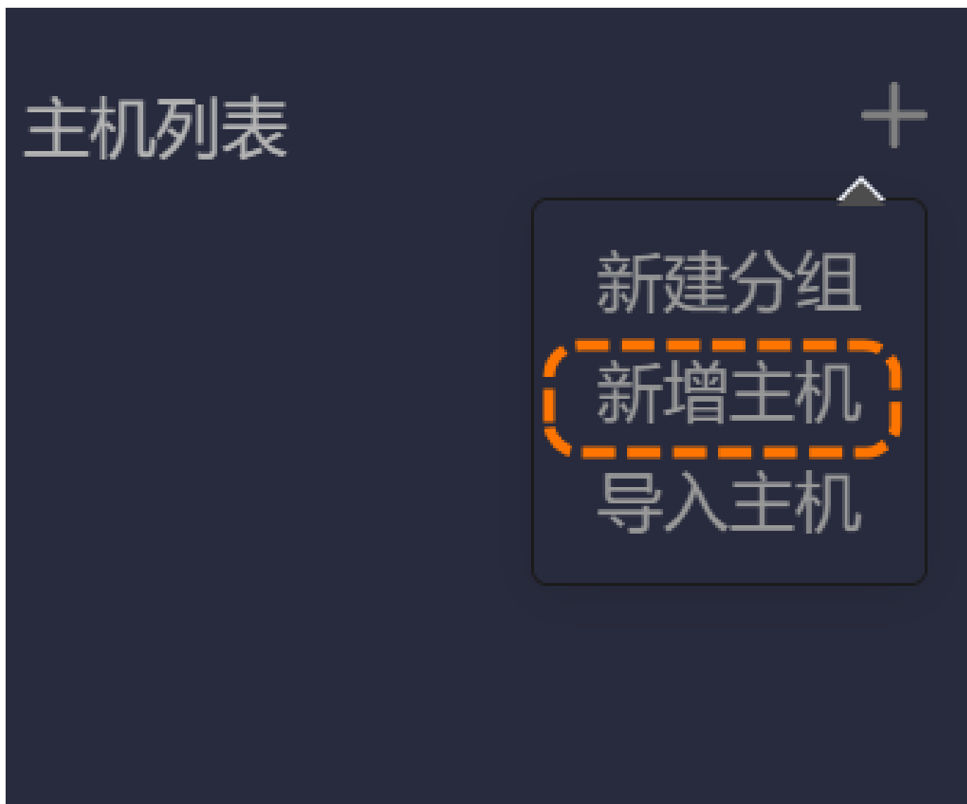
图 11-13 新增主机
