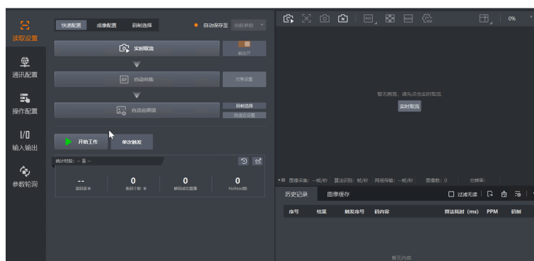
图 8-6 条码裁剪
