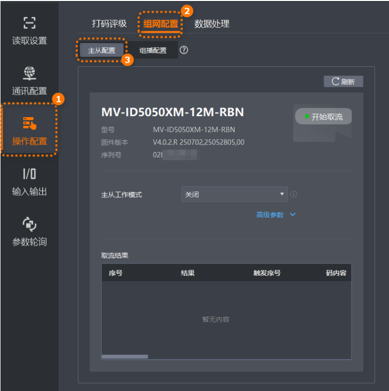
图 9-2 主从配置
