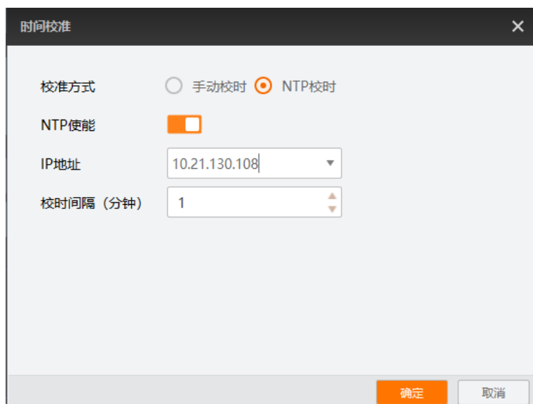
图 6-15 NTP 校时
